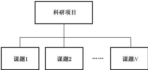
图 2 无子项目的科研项目与科研课题关系图
